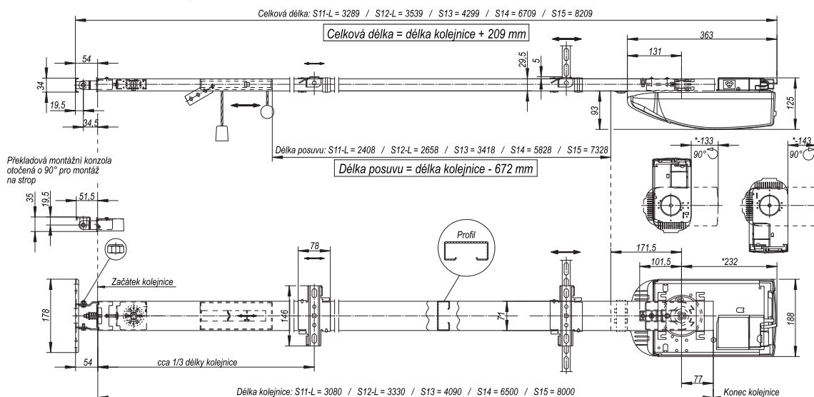
Tabulka použitelnosti jednotlivých délek kolejniček pro sekční vrata DELTA a PRAKTIK
