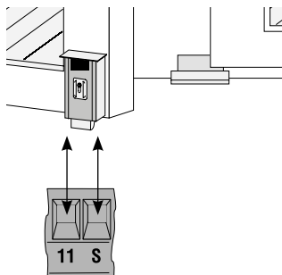
Připojení elektrického zámku (max. 12 V – 15 W)
