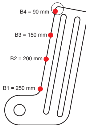
DETAIL: B
