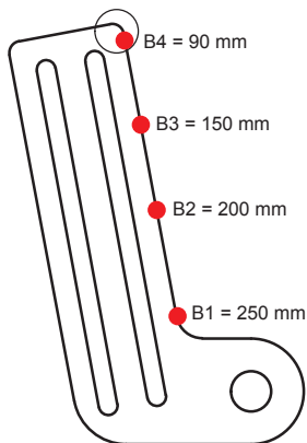
DETAIL: B
